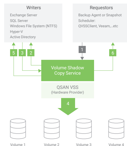
Интеграция с Volume Shadow Copy Service
