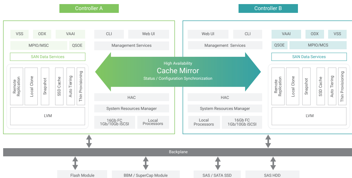
Архитектура ОС QSAN SANOS
